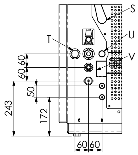
DETTAGLIO A
